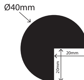
RCAP40X40W
