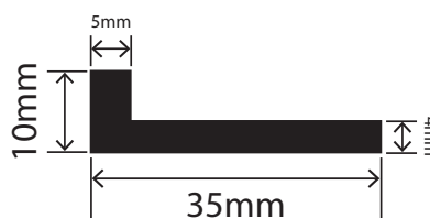
RCAP35X10VE
