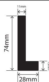
RCAP28X74W
