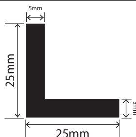
RCAP25X25L
