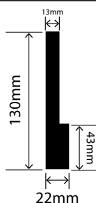
RCAP22X130W
